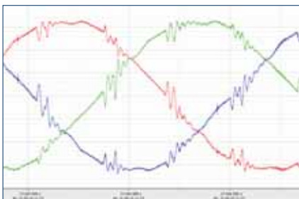
Abb. Grafik 1: Spannungskurvenformen an der NSHV vor der Installation des hybriden Power Conditioners: Beim Antrieb großer Gleichstrommaschinen verursachen Thyristor-Stromrichter die Einbrüche. Erkennbar sind zwei kurz hintereinander auftretende Einbrüche von zwei unabhängig gesteuerten Brecherantrieben inklusive mehrfacher Nulldurchgänge sowie starke resonante Nachschwinger.
